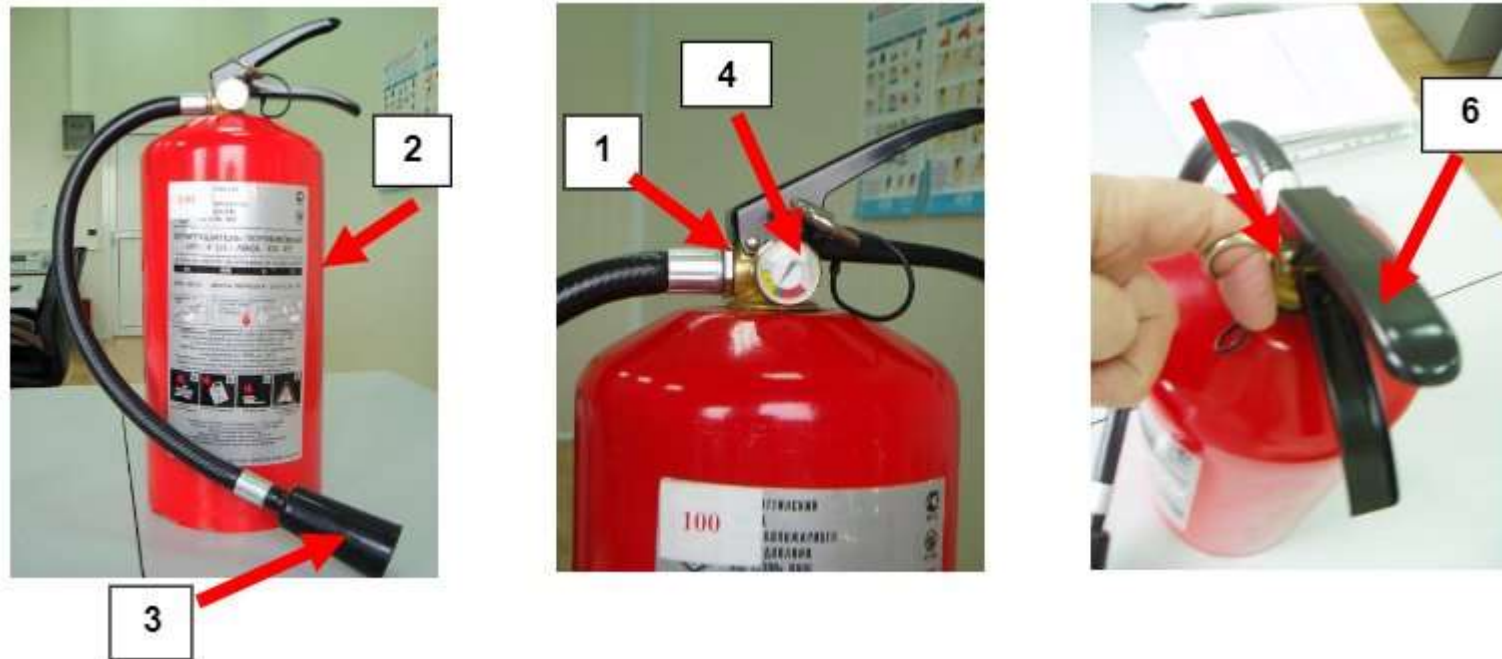
Рис.1. Порошковый огнетушитель типа ОП-4(з)
